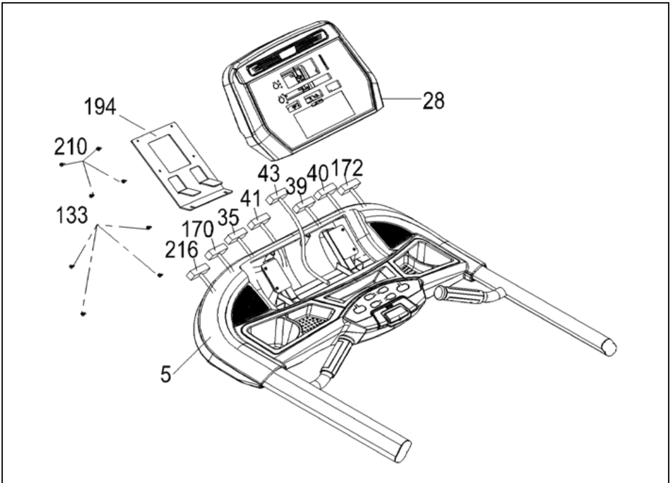
Benötigte Teile für Schritt 2 Needed parts for Step 2
